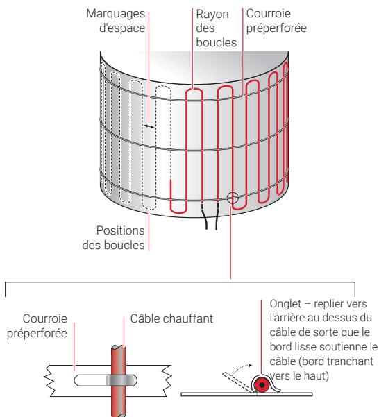
Figure 29 : Disposition du câble à l'aide de courroies préperforées
