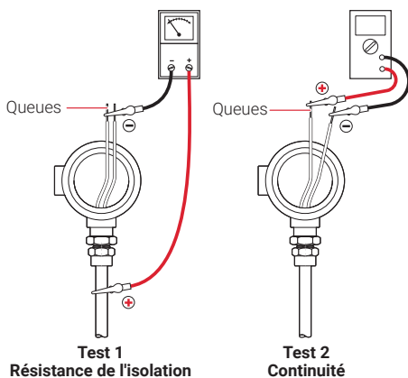
Figure 32 : Branchez le mégohmmètre et le multimètre.
