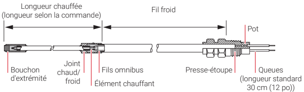
Figure 2 : Vue en coupe du câble à isolation minérale XMI-A de conception D
