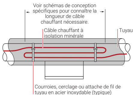
Figure 22 : Support de type patin et manchon
