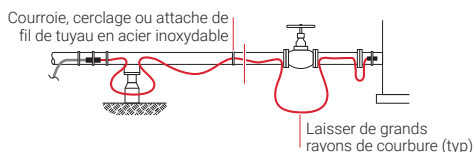
Figure 13 : Allocations pour vannes, brides, et supports de tuyau
