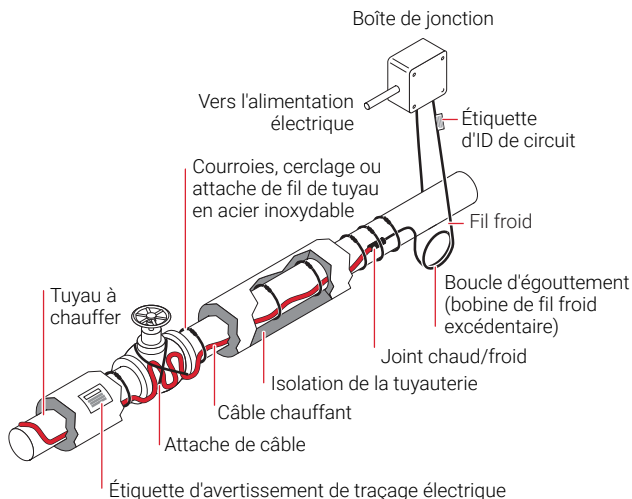
Figure 1 : Système type de conception B
