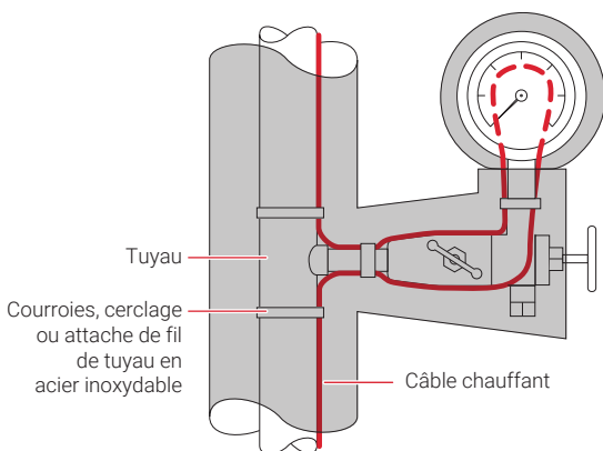
Figure 27 : Manomètre
