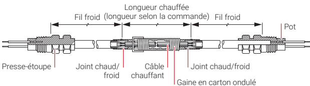
Figure 4 : Vue en coupe du câble à isolation minérale XMI-L de conception E
