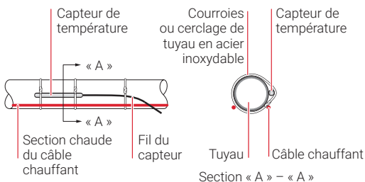
Figure 28 : Capteur de température monté sur le tuyau
