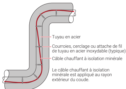
Figure 19 : Installation au niveau du coude à 90°
