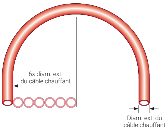
Figure 9 : Rayon de cintrage minimal
