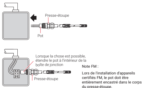
Figure 31 : Raccordement de la boîte de jonction
