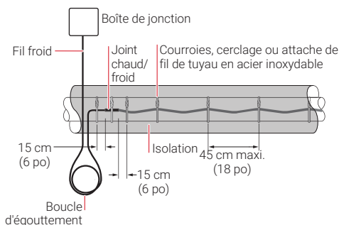
Figure 16 : Espacement de la courroie pour tuyaux
