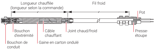
Figure 3 : Vue en coupe du câble à isolation minérale XMI-L de conception D
