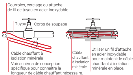
Figure 17 : Fixation de plusieurs longueurs de câble
