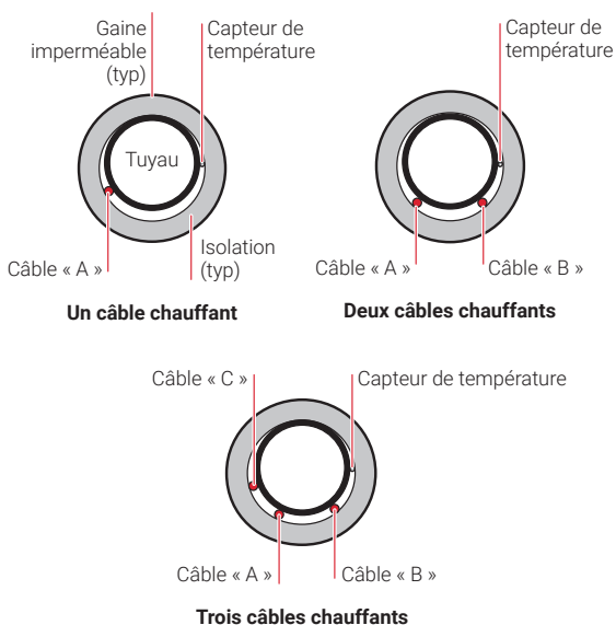
Figure 8 : Positionnement du câble – coupe transversale
