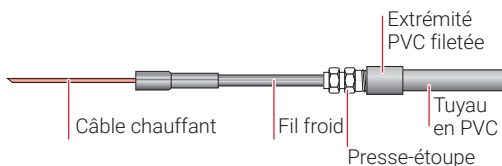
Figure 7 : Protection des extrémités du fil froid
