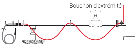
Figure 12 : Fixation du raccord chaud/froid et du capuchon d'extrémité
